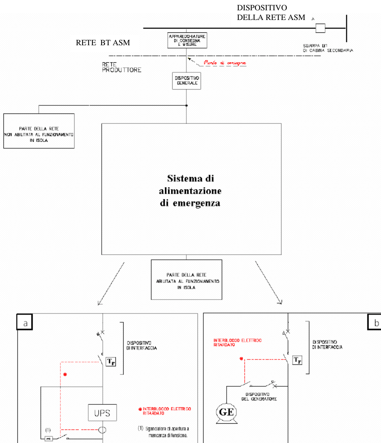
Figura 3 - Schema di base del collegamento di un gruppo di alimentazione di emergenza connesso alla rete ASM previsto per il funzionamento in regime breve di parallelo. a) UPS; b) gruppo elettrogeno.
